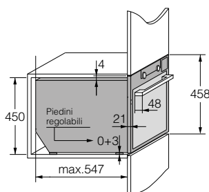
Vista laterale
