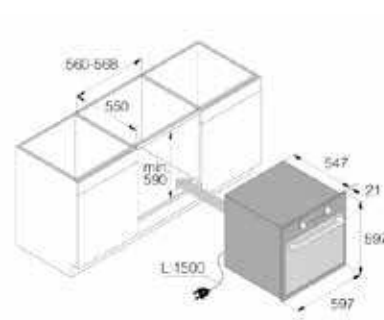
Installazione sottopiano
