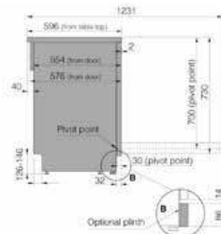
Vista laterale
