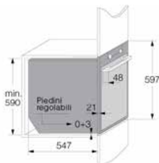
Vista laterale
