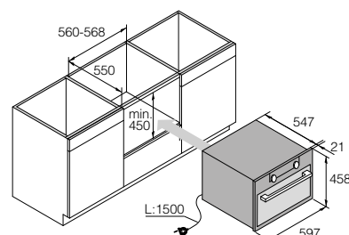
Installazione sottopiano
