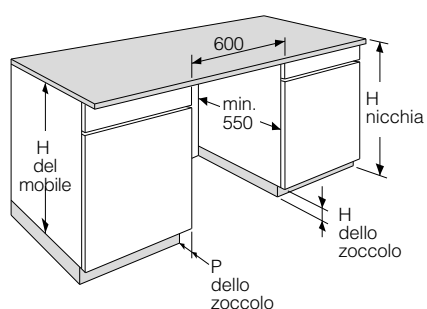
Dimensioni nicchia
