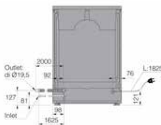
Vista posteriore
