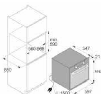
Schema d'installazione
