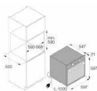
Schema d'installazione
