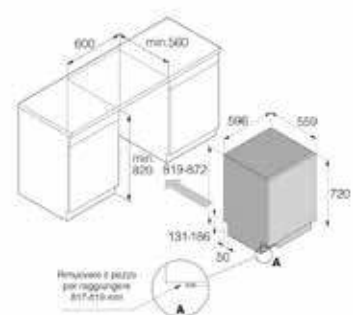
Dimensioni di incasso
