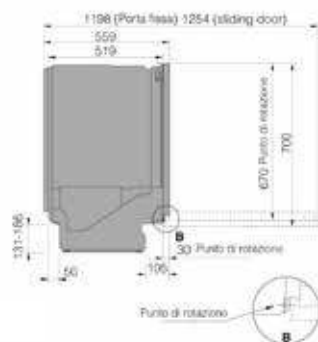
Vista laterale
