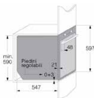
Vista laterale
