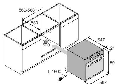
Installazione sottopiano
