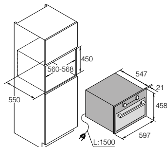
Schema d'installazione
