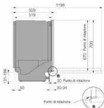
Vista laterale
