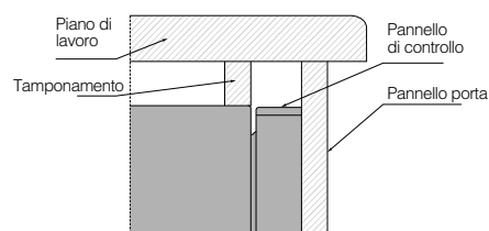
Installazione speciale
