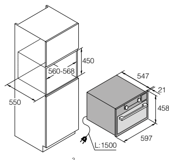
Schema d'installazione
