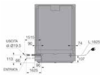
Vista posteriore
