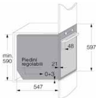
Vista laterale
