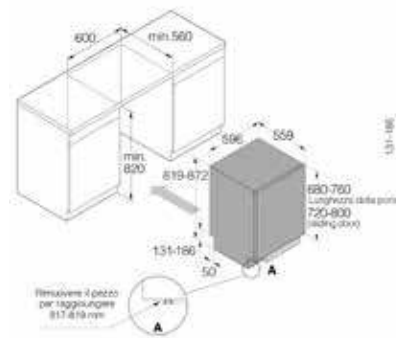
Dimensioni di incasso
