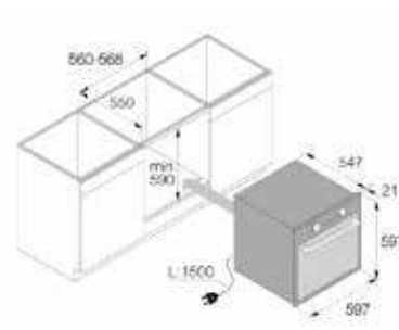
Installazione sottopiano
