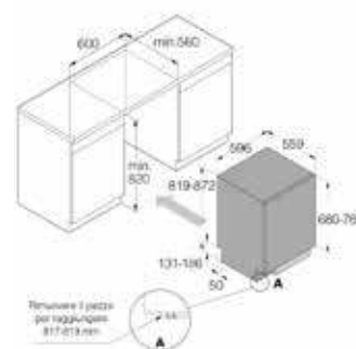
Dimensioni di incasso
